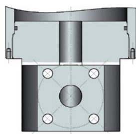
Beispiel 2: radialer Flanschanschluss
