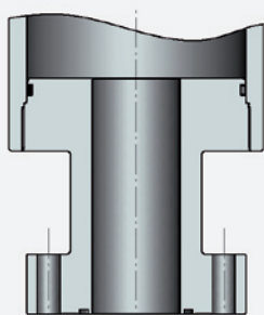
Beispiel 3: axialer Flanschanschluss
