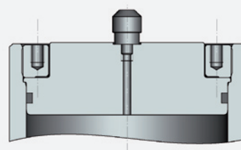
Beispiel 1: Füllventil für Membranspeicher M 28 x 1,5
