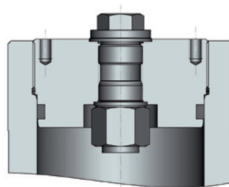
Beispiel 3: BSD-Gas-Füllventil Anschluss 3/4"
