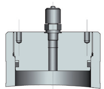
Beispiel 3: Minimess-Füllventil M 16 x 1,5
